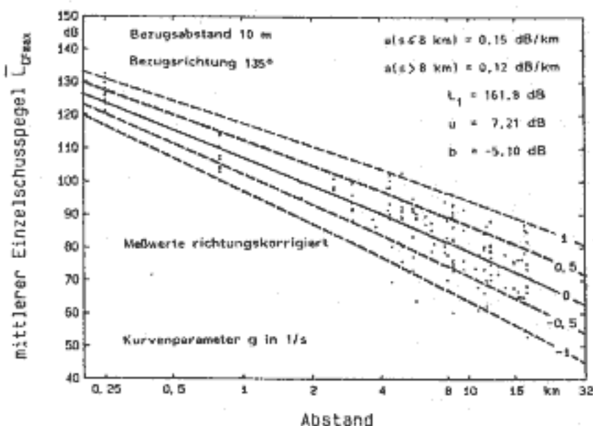
Abb. 3: Abstandsabhängigkeit des C- und FAST-bewerteten mittleren Maximalpegels des Mündungskalles von Panzerkanonen
