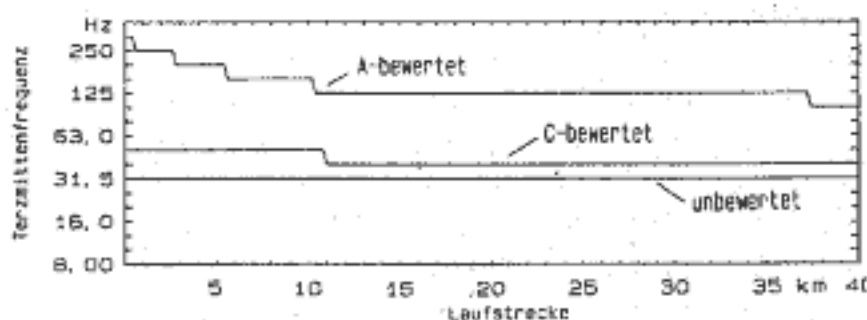
Abb. 2: Abstandsabhängigkeit der pegelbestimmenden Terz des Mündungskalles von Panzern für drei Bewertungsarten
